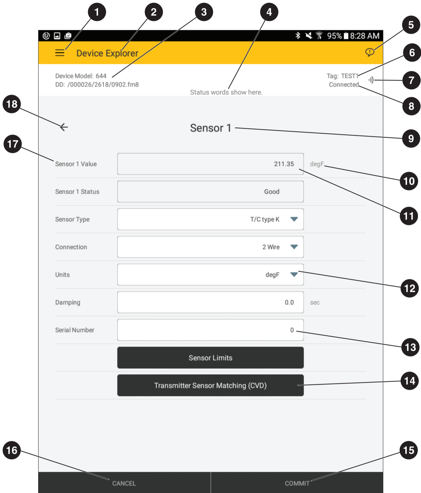
그림 1. 샘플 메뉴
