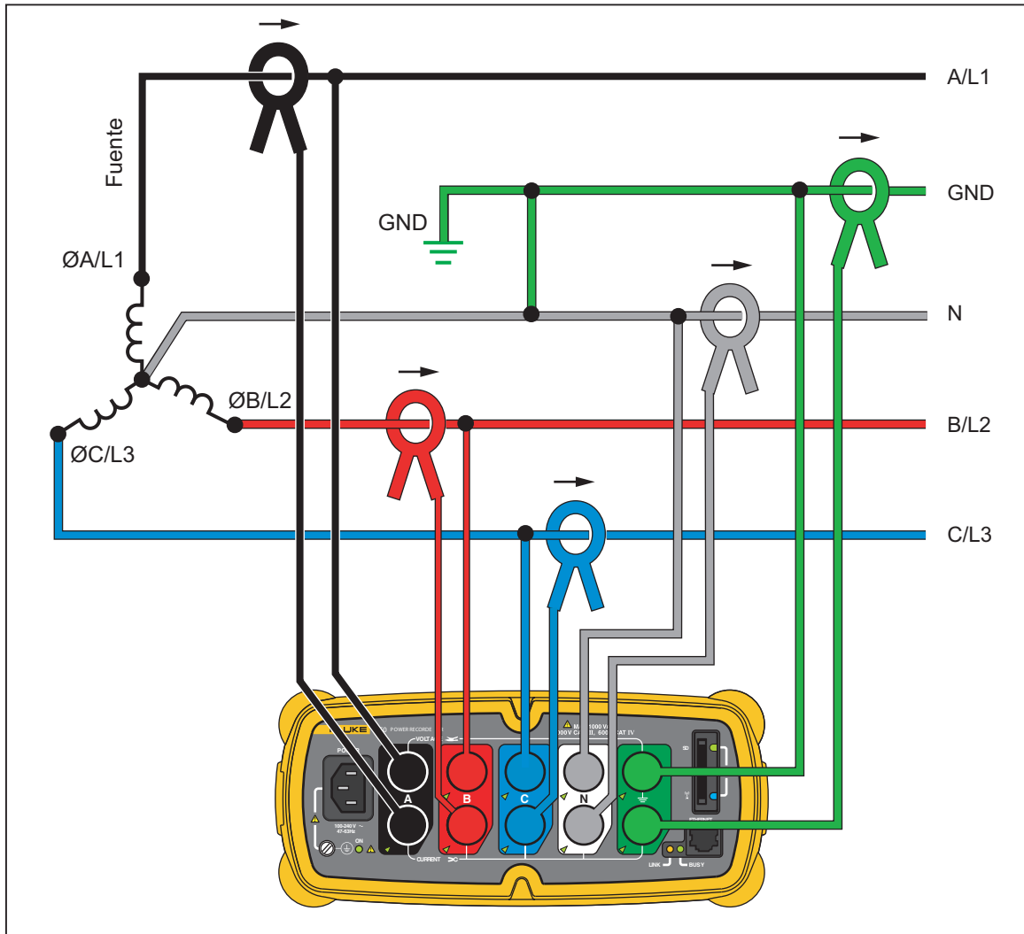
Figura 7. Estrella trifásico
