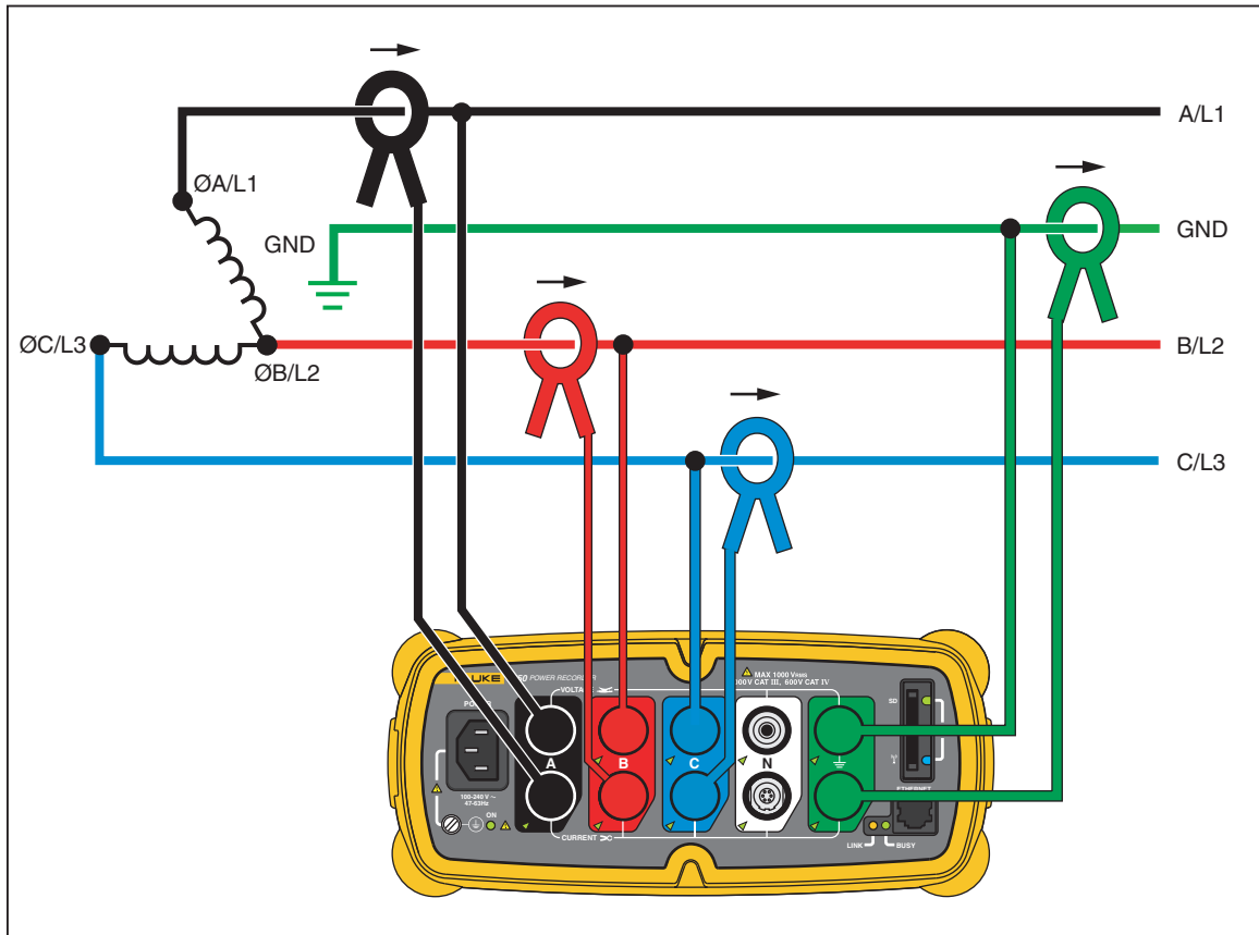
Figura 11. Patilla abierta trifásico
