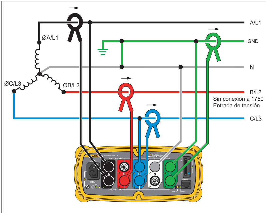
Figura 13. Estrella de 2 ½ elementos
