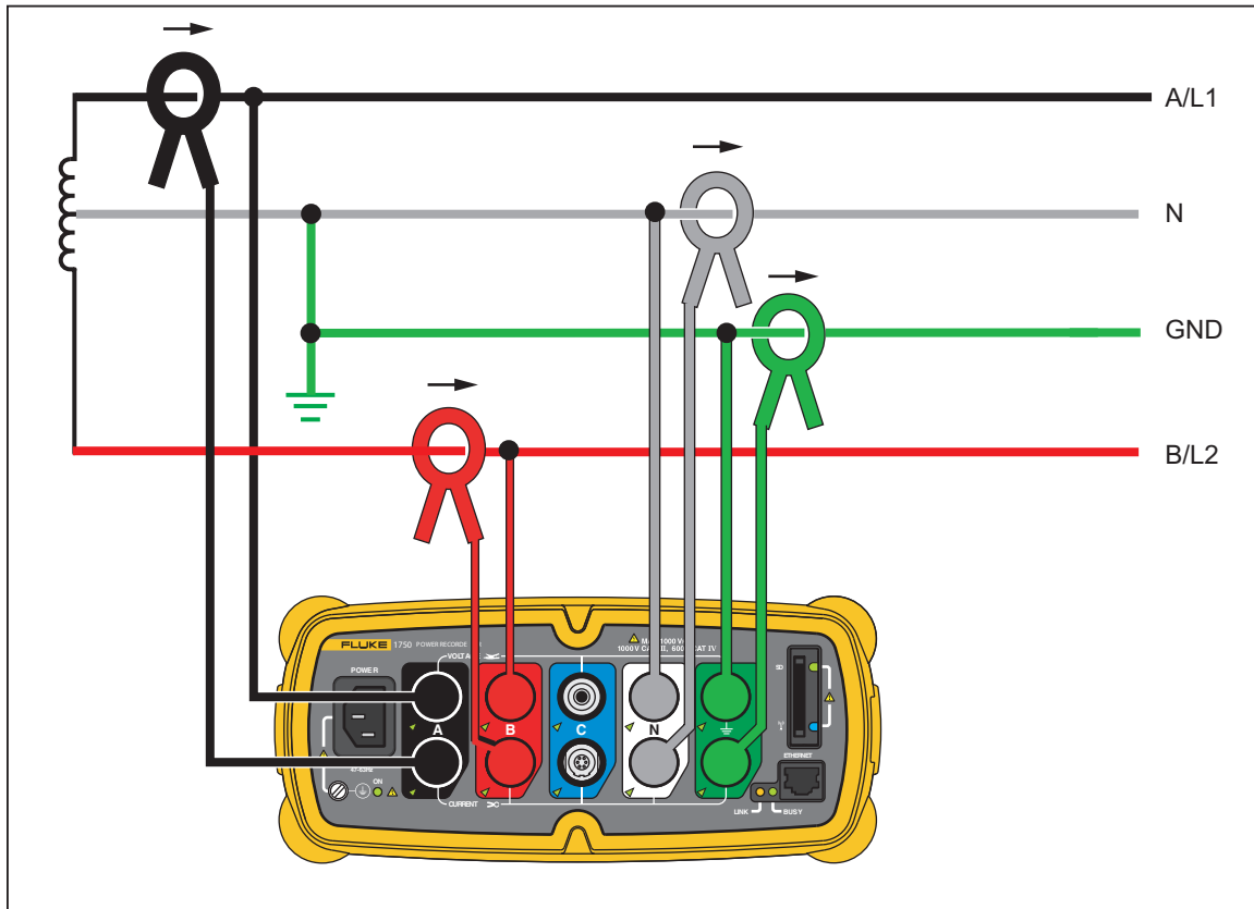
Figura 6. Monofásico-fase dividida
