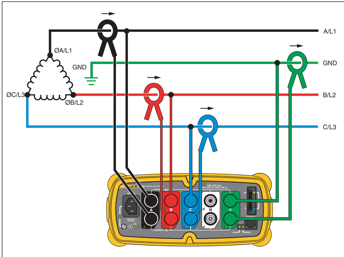
Figura 8. Triángulo trifásico
