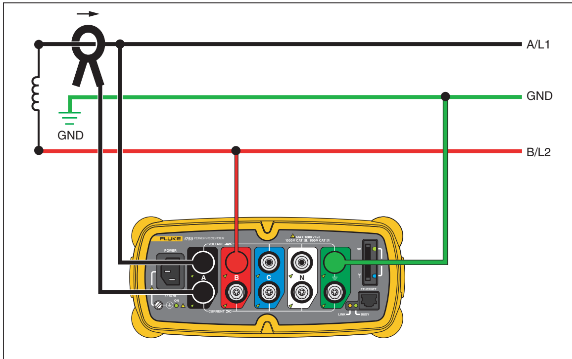
Figura 5. TI monofásico sin neutro
