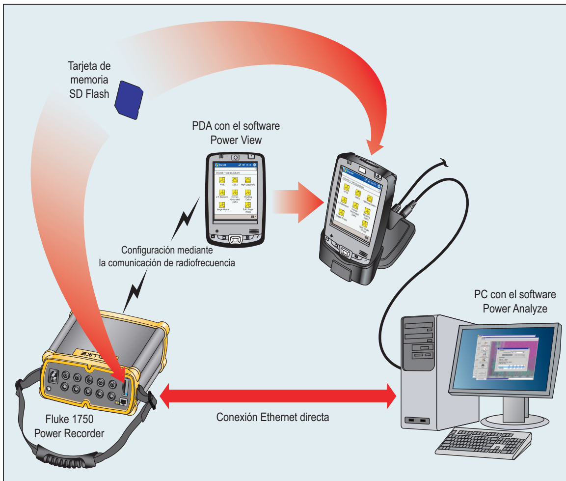
Figura 14. Conexión con el registrador
