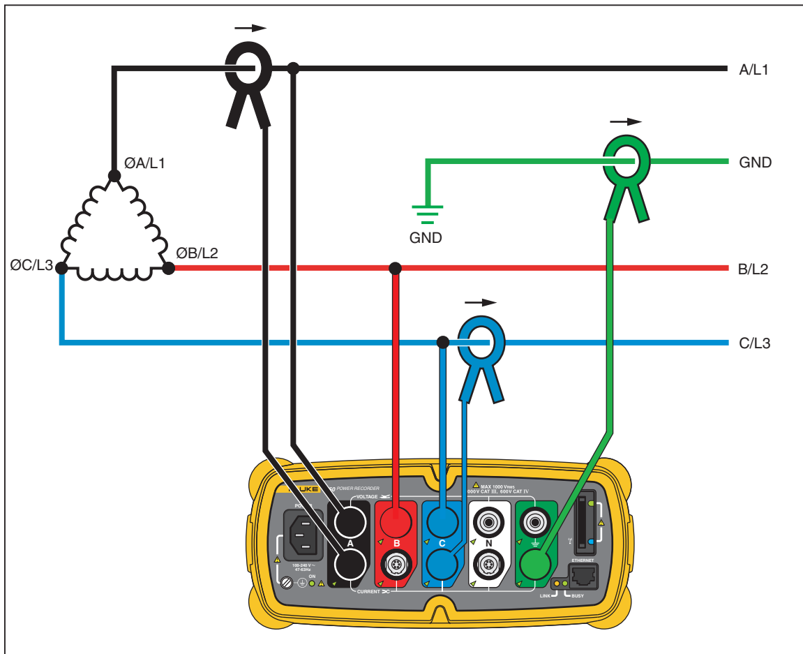
Figura 12. Triángulo de dos elementos
