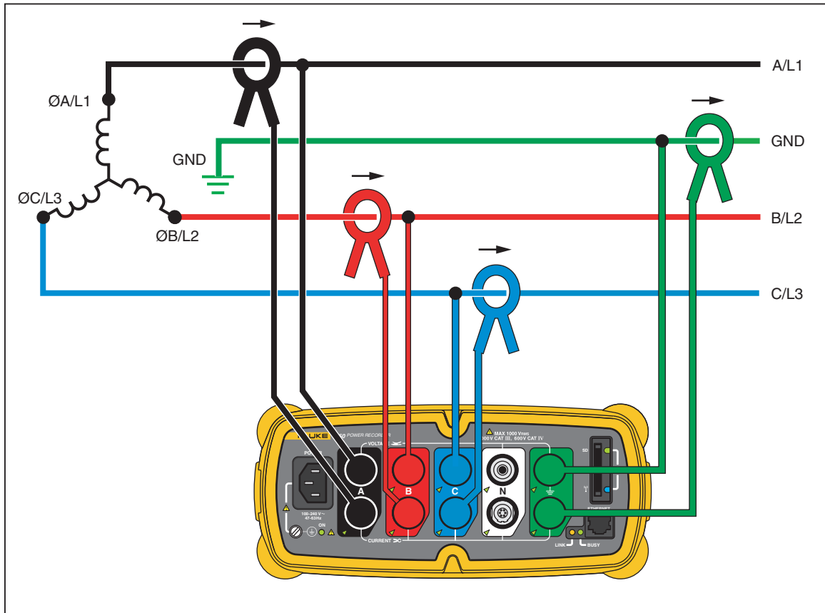
Figura 9. TI trifásico
