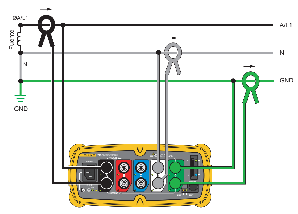
Figura 4. Monofásico más neutro
