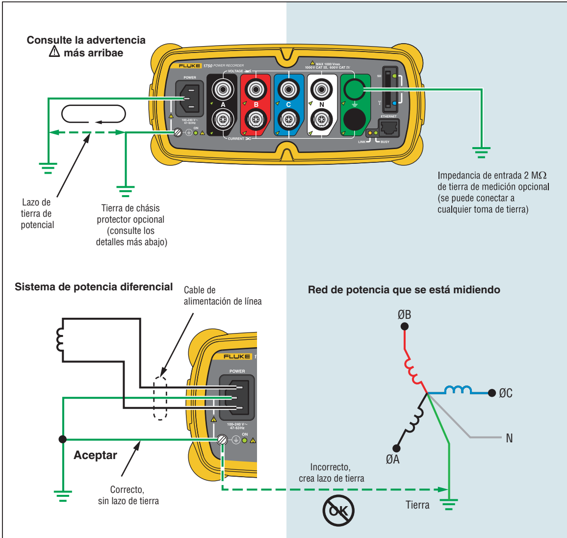
Figura 3. Conexión del terminal de tierra auxiliar
