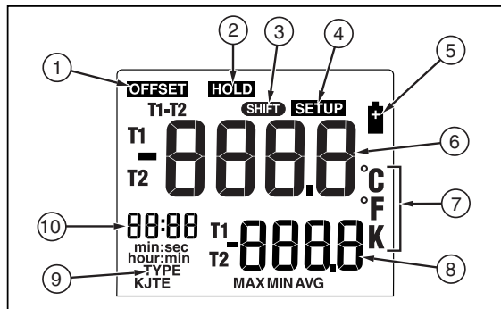
그림 2. 디스플레이 구성요소
